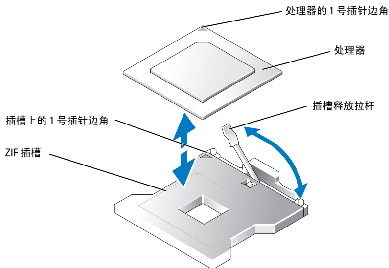
图 1-2. 装卸处理器
