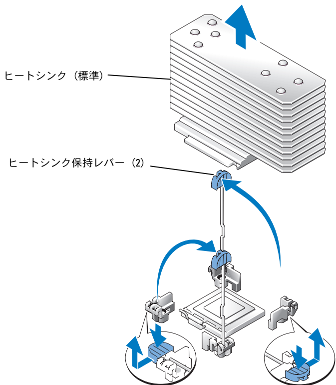
図 1-1 ヒートシンクの取り外しと取り付け
