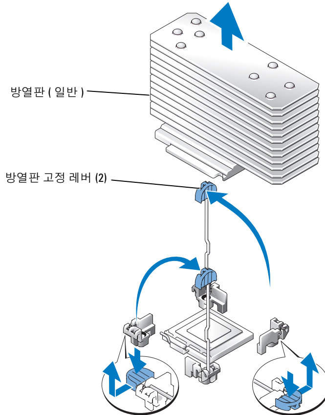
그림 1-1. 방열판 제거 및 설치
