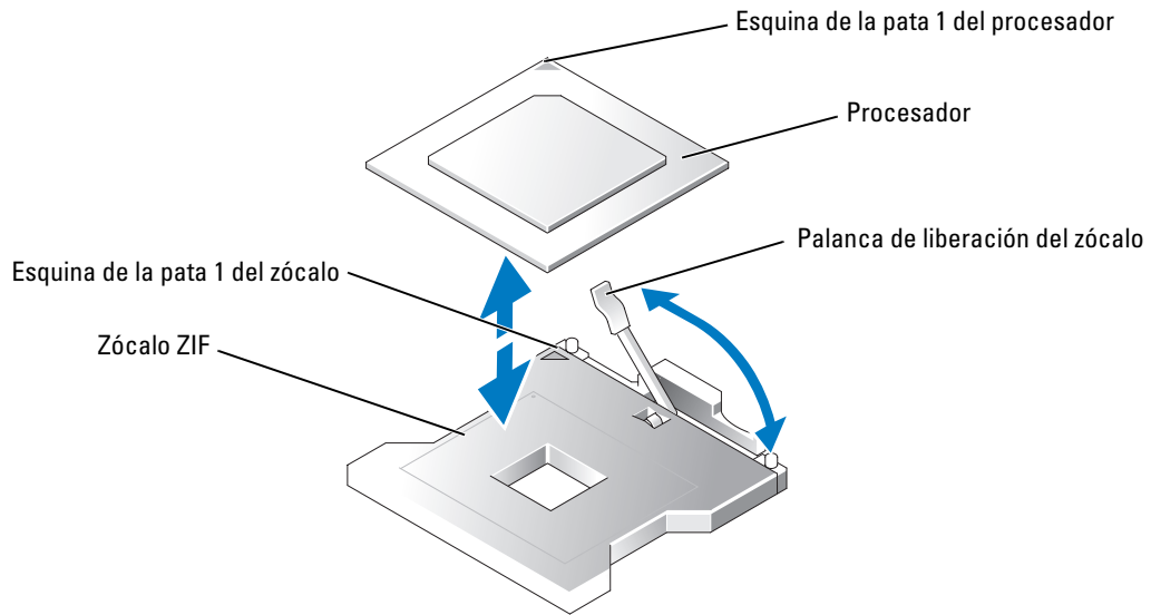
Figura 1-2. Extracción e instalación del procesador
