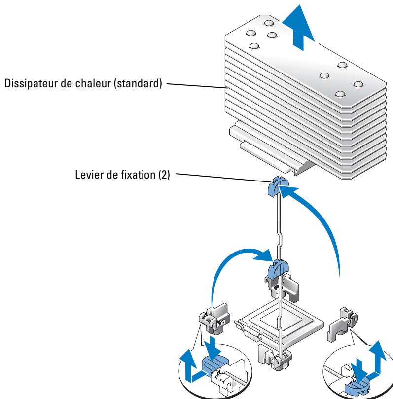
Figure 1-1. Retrait et installation du dissipateur de chaleur
