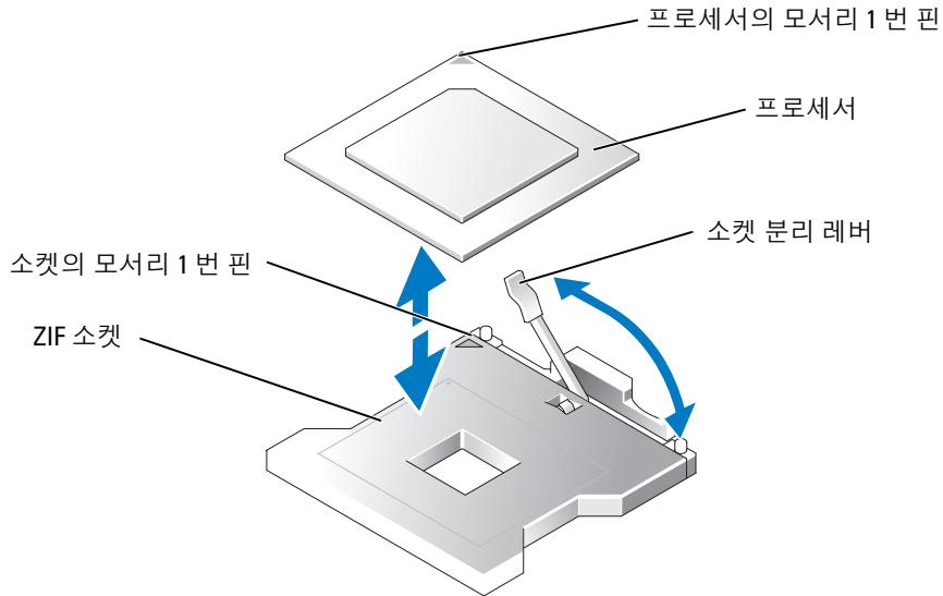
그림 1-2. 프로세서 제거 및 설치
