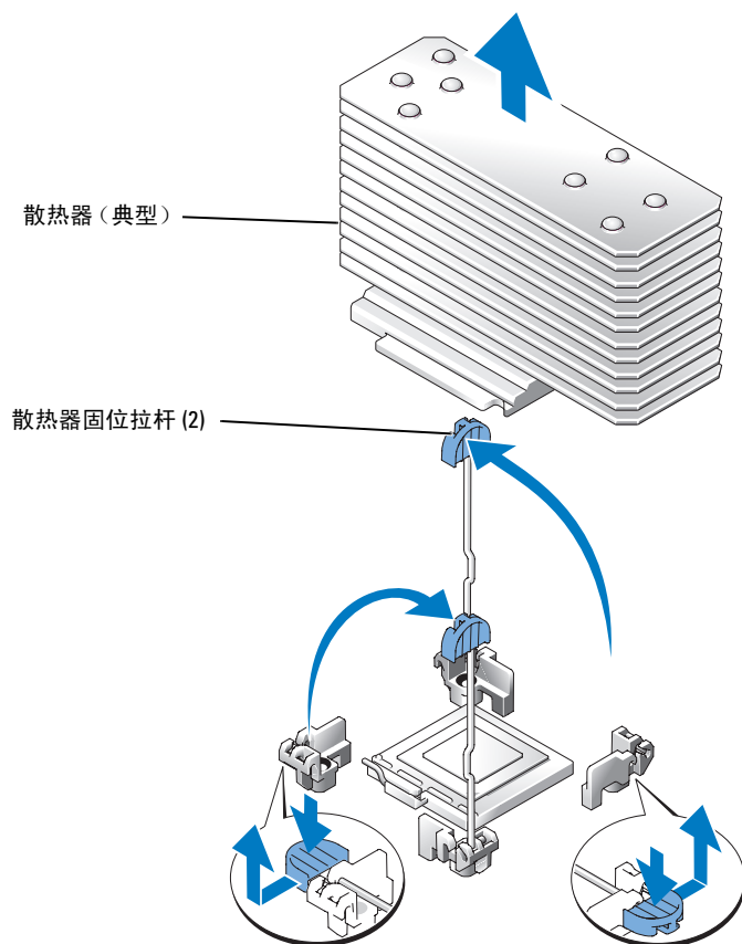
图 1-1. 装卸散热器
