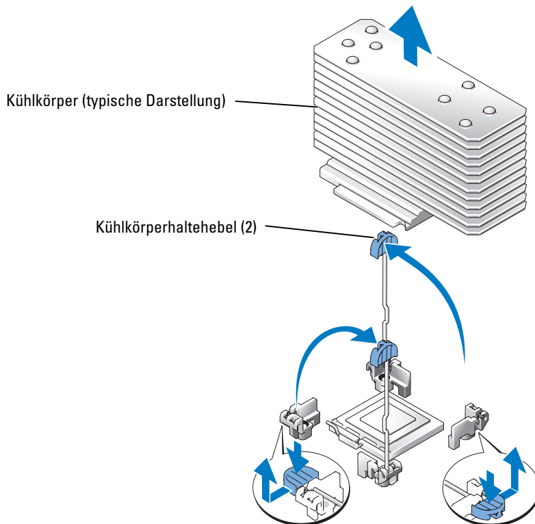
Abbildung 1-1. Kühlkörper entfernen und installieren
