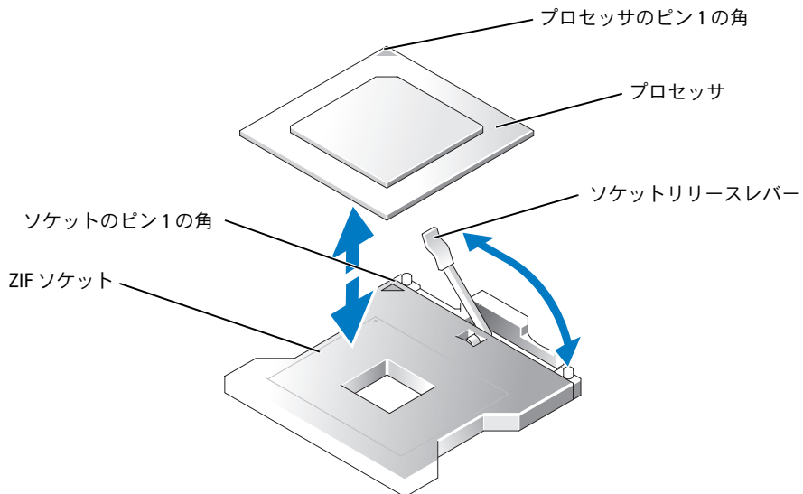
図 1-2 プロセッサの取り外しと取り付け
