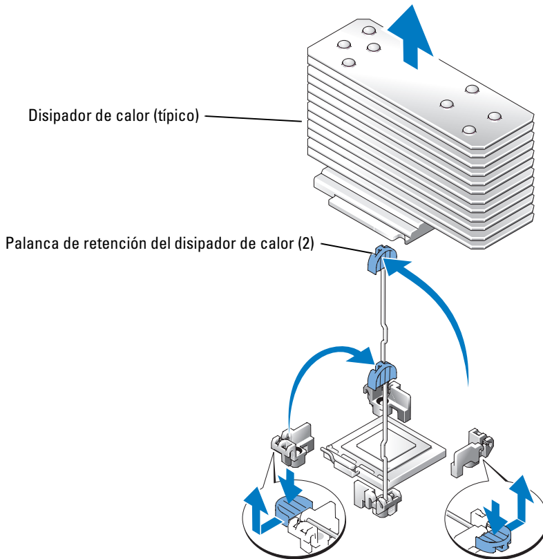
Figura 1-1. Extracción e instalación del disipador de calor
