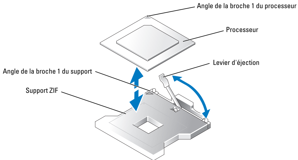
Figure 1-2. Retrait et installation du processeur
