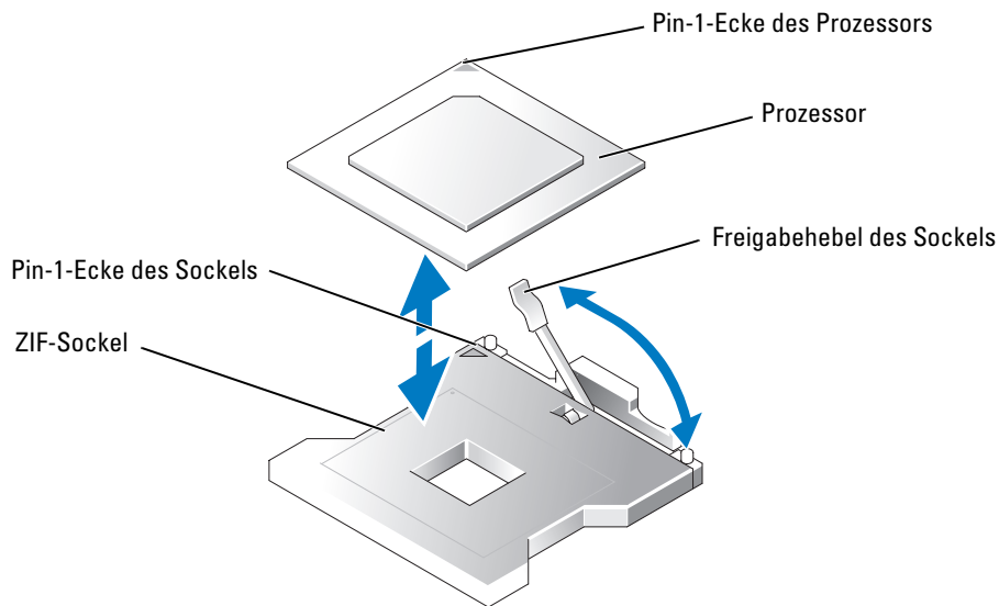
Abbildung 1-2. Prozessor entfernen und installieren
